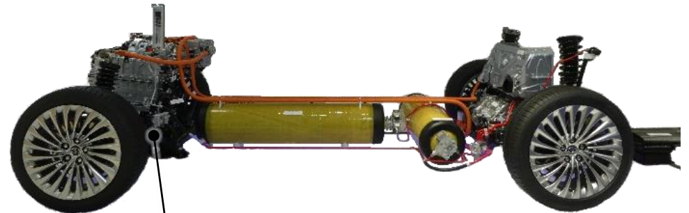
トヨタFCスタック (燃料電池)
