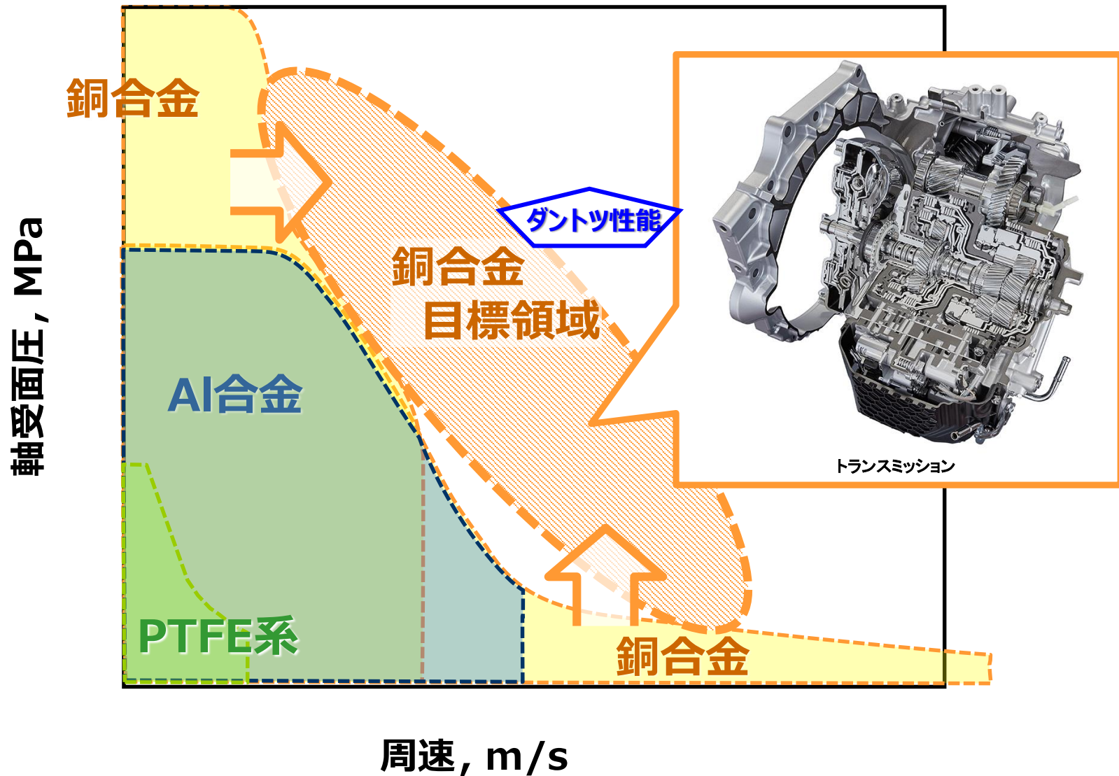
《ブシュ材料の適用可能範囲（流体潤滑）》
