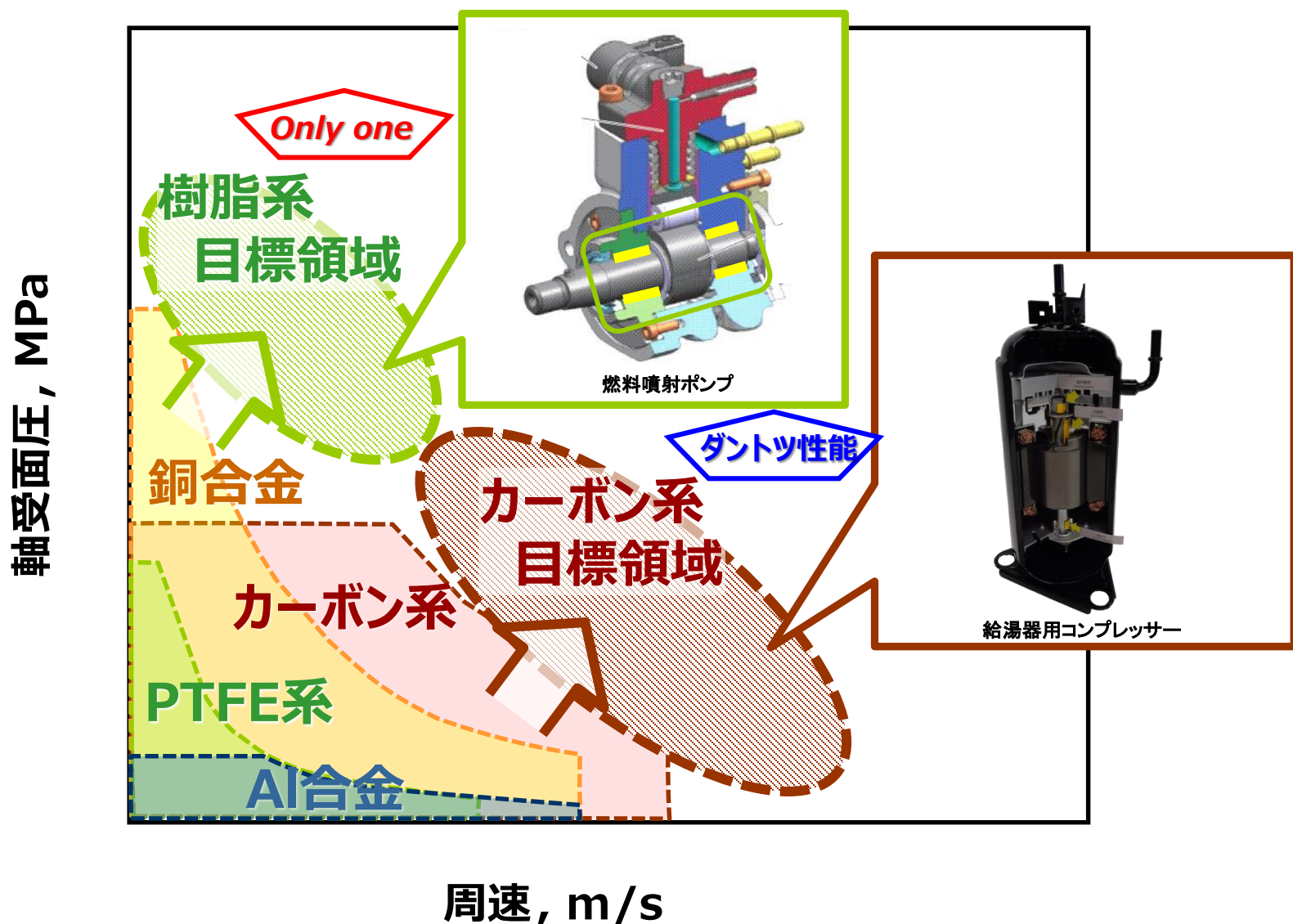
《ブシュ材料の適用可能範囲（境界潤滑～混合潤滑領域）》
